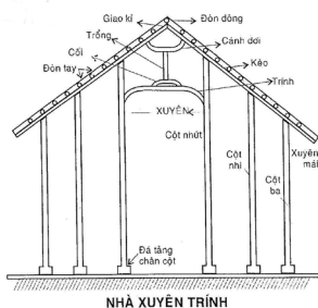
Một vĩ nhà xuyên trính
